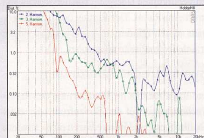
Im Gruntbereich höhere, mit zunehmender Frequenz sehr gleichmäßig abfallende Verzerrungen.
