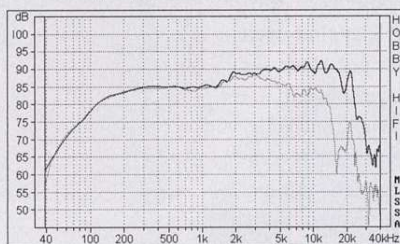
Überragende Linearität und Breitbandigkeit.
