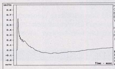
Äußerst schnelles Ein- und Ausschwingen.
