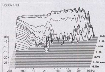
Exzellentes transientes Verhalten, leichte Resonanzstörung in den Mitteln.
