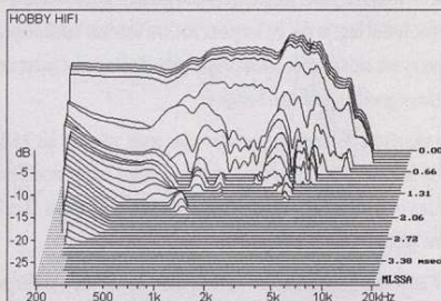
Gleichmäßiges schnelles Ausschwingen, minimaler Resonanzanflug bei 1 kHz.
