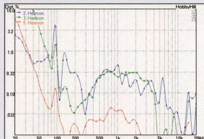
Niedrige Klirrwerte.
