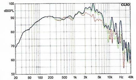
Frequenzgang für 0/15/30
