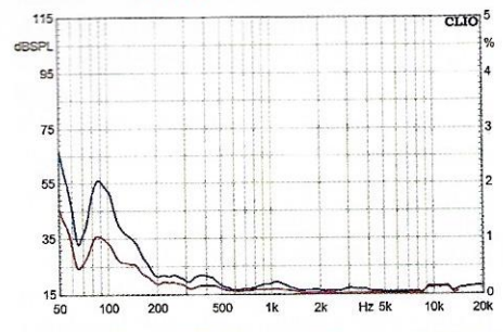
Klirrfaktor K2/K3 für 95 dB/1 m
