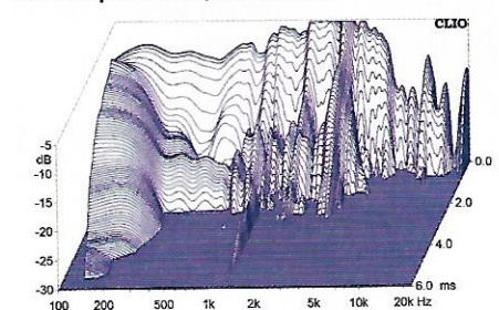
Zerfallspektrum (Wasserfall)
