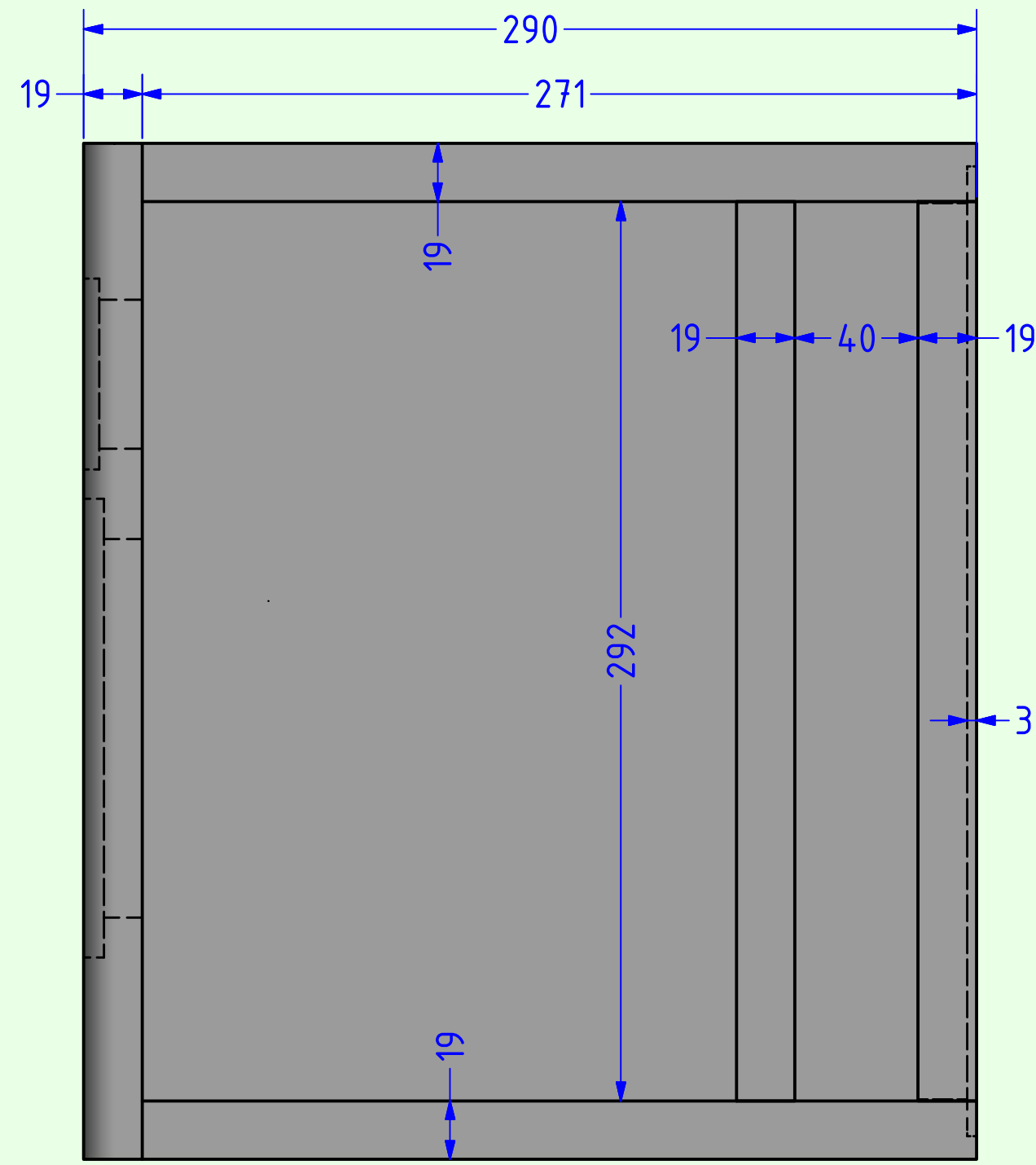
Seitenansicht (ohne rechte Seitenwand)
