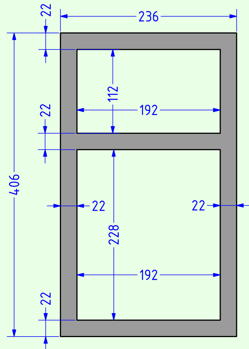
Versteifungsrahmen
