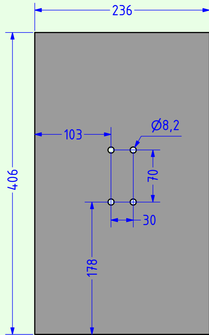
Rückwand
