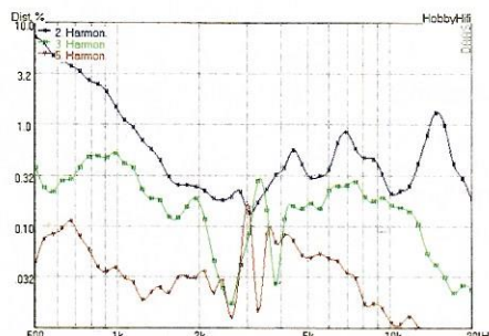
Klirrfaktor-Frequenzgänge K2, K3 u. K5 bei 90 dB mittlerem Schalldruckpegel Im unteren Hochtönenbereich besonders niedriger, zu höheren Frequenzen etwas ansteigender Klirr.
