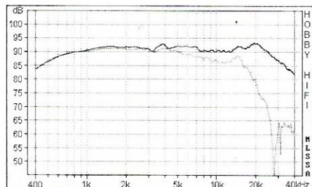
Schalldruck-Frequenzgang auf unendlicher Schallwand axial und unter 30° Exzellente Linearität, Ausgewogenheit und Breitbandigkeit.
