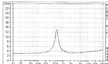
Impedanz-Frequenzgang Sehr niedrige Resonanzfrequenz, sauber ausgeprägtes Resonanzmaximum.
