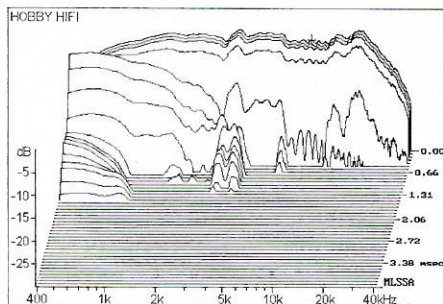
Wasserfallpektrum auf unendlicher Schallwand axial Hervorragend schnelles und gleichmäßiges Ausschwingen trotz minimaler Artefakte um 4 kHz.
