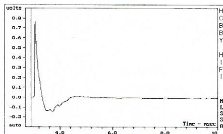
Sprungantwort auf unendlicher Schallwand axial Bestens kontrolliertes Ein- und Ausschwingen.
