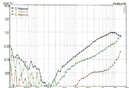
Klirrfaktor K2, K3 und K5 über Signalpegel bei 1,5 kHz Hervorragende Pegelfestigkeit, im Kleinsignalbereich leicht erhöhter Klirr.
