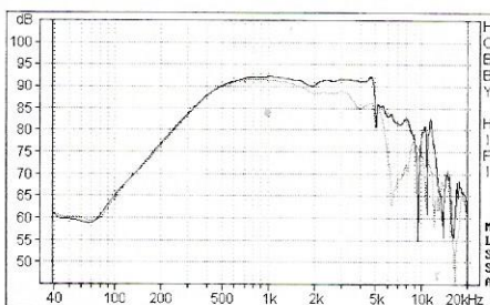
Schalldruck-Frequenzgang in unendlicher Schallwand axial und unter 30° Ideal ausgewogen und linear, scharfe Abrisskante bei 5 kHz.
