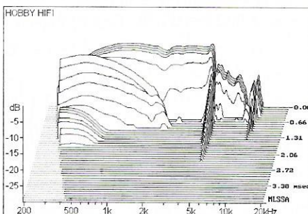
Wasserfallspektrum in unendlicher Schallwand axial Resonanzstelle bei 5 kHz mit langem Nachschwingen, darunter fehlerfrei.
